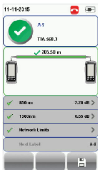
Результаты автоматического тестирования оптического волокна MMEF
